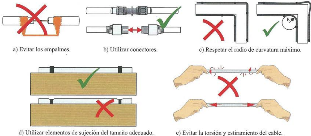
Figura 6.86. Normas básicas de instalación.
