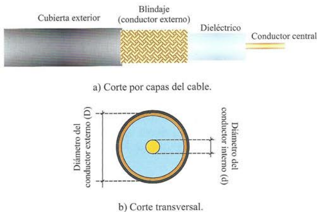
Figura 6.7. Estructura del cable coaxial.
