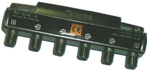
Figura 6.17. Derivador de cuatro salidas.
