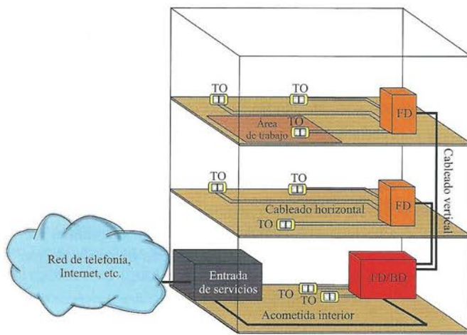
Figura 6.42. Ejemplo de cableado estructurado en varios edificios.
