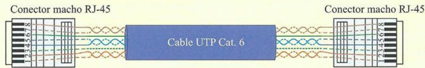
Figura 6.90. Cable de conexión directa.
