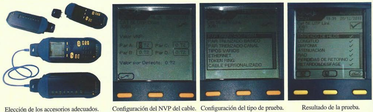
Figura 6.60. Certificación de un latiguillo de conexión.
