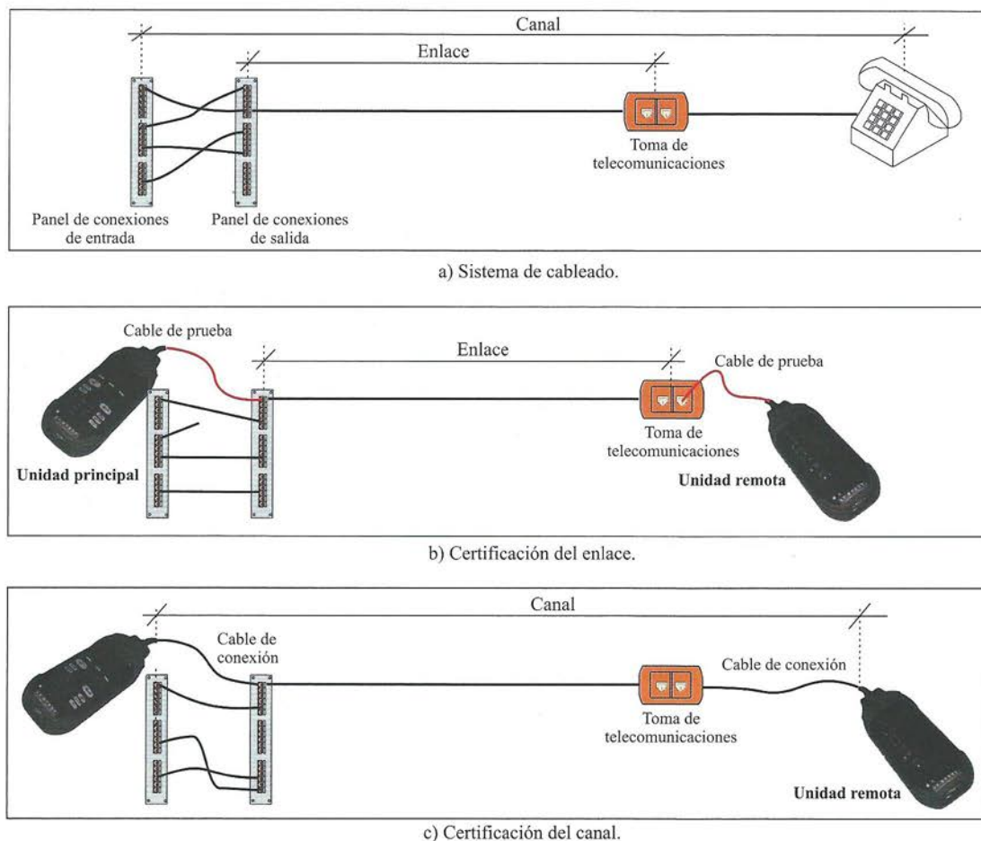
Figura 6.50. Certificación de una instalación.
