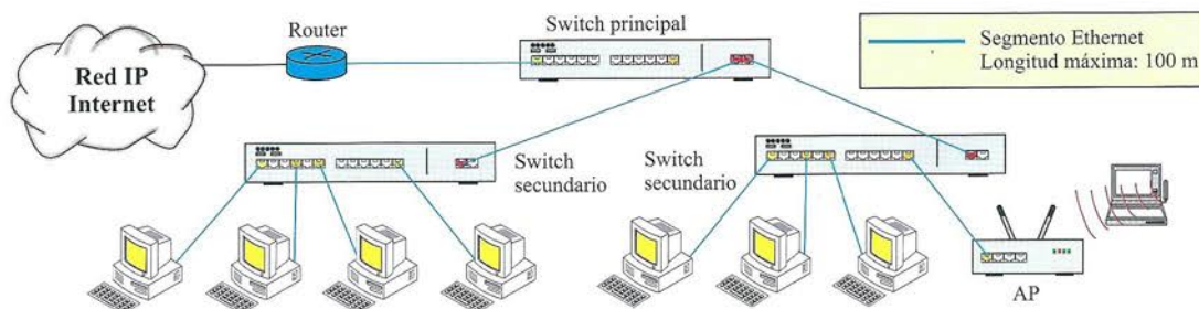
Figura 6.37. Red de datos de tecnología Ethernet.
