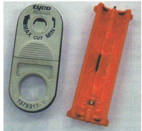
Figura 6.12. Peladora de cable.
