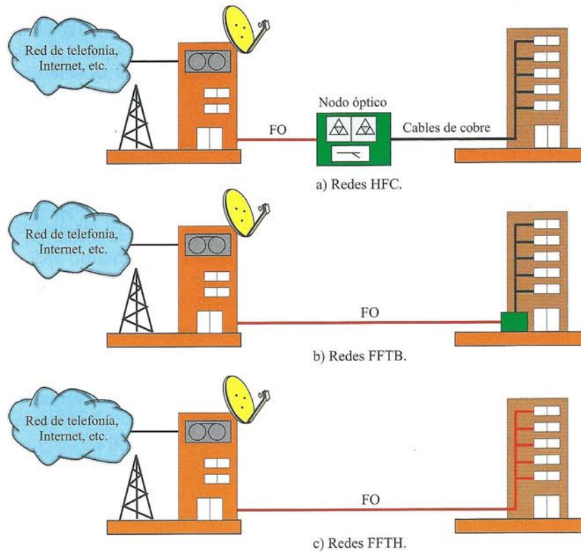
Figura 6.3. Estructura simplificada de las redes de acceso de fibra óptica.
