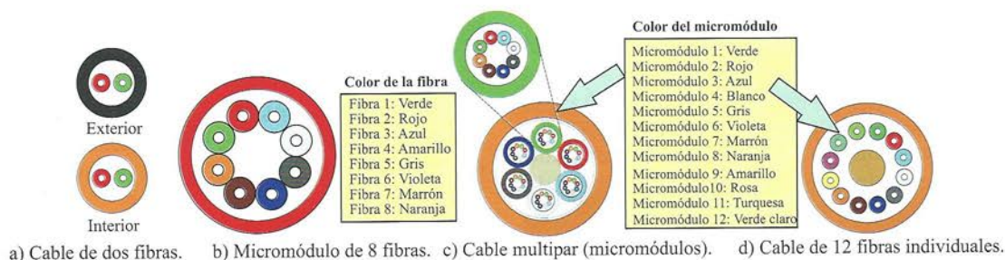
Figura 6.83. Identificación de fibras ópticas.
