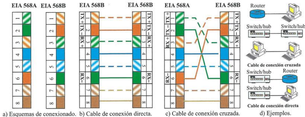
Figura 6.41. Esquemas de conexionado.
