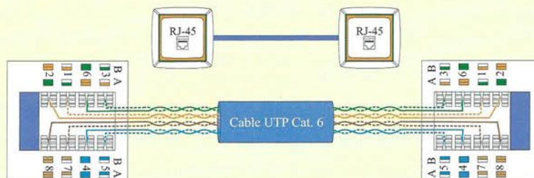
Figura 6.89. Cableado fijo de una instalación.
