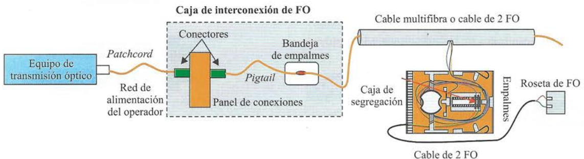
Figura 6.78. Red de distribución de FO.
