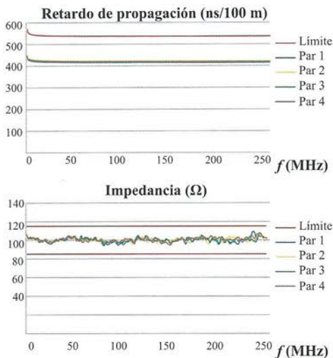
Figura 6.56. Ejemplo de resultados de medida de una instalación.
