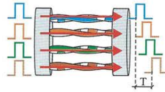
Figura 6.51. Retardo diferencial.
