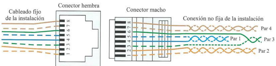
Figura 6.32. Cableado típico de un conector RJ-45.
