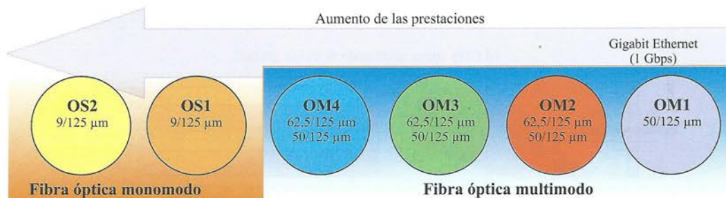
Figura 6.68. Prestaciones de la fibra óptica en relación a su clasificación.
