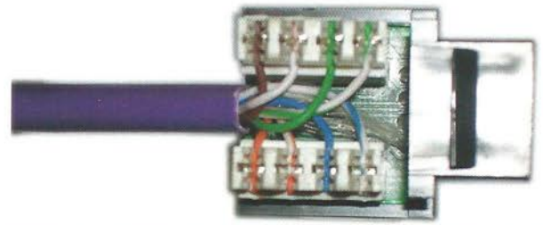
Figura 6.33. Conexión del cableado de par trenzado.
