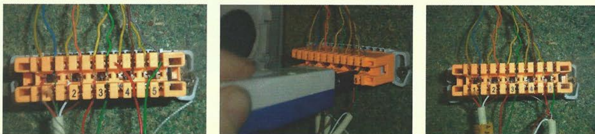
Figura 6.27. Conexión del cable de pares en una regleta.
