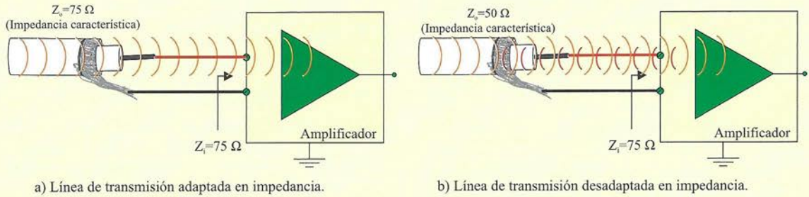
Figura 6.9. Comunicación entre dos equipos con cable coaxial.
