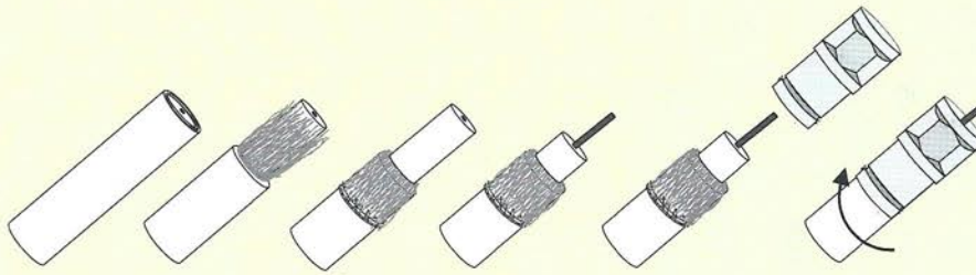
Figura 6.14. Realización de una conexión de cable coaxial con un conector tipo F.
