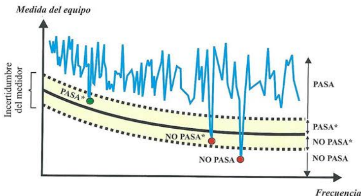
Figura 6.58. Certificación de una red: resultado pasa/no pasa.
