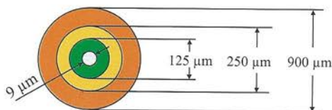
Figura 6.66. Estructura típica de un cable de fibra óptica.
