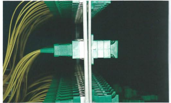
Figura 6.79. Paneles de conexión de fibra óptica.
