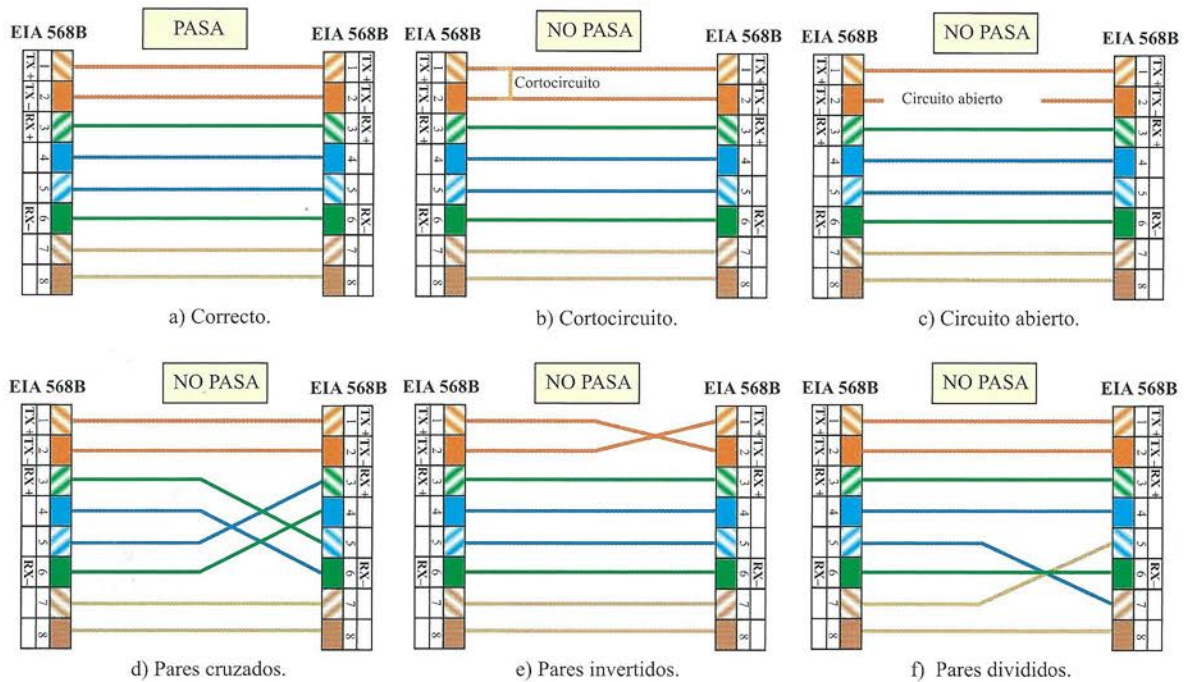
Figura 6.48. Errores típicos en el mapeado de un cable de pares trenzados.
