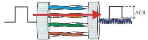
Figura 6.55. ACR.
