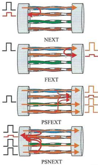
Figura 6.54. Parámetros relacionados con la diafonía.
