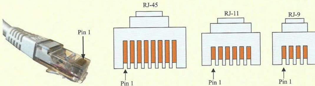
Figura 6.94. Conectores RJ.
