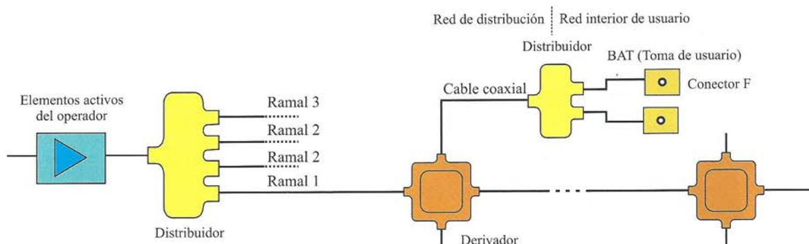
Figura 6.15. Ejemplo de red de distribución de la señal de cable coaxial.
