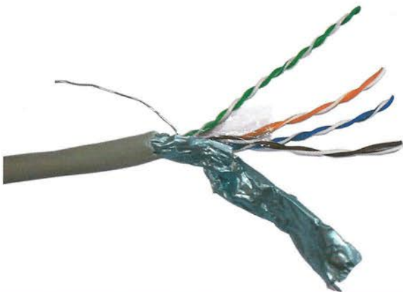
Figura 6.30. Cable FTP.
