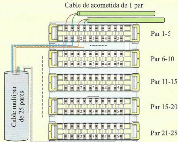
Figura 6.88. Conexión de un cable de pares en las regletas de conexión.
