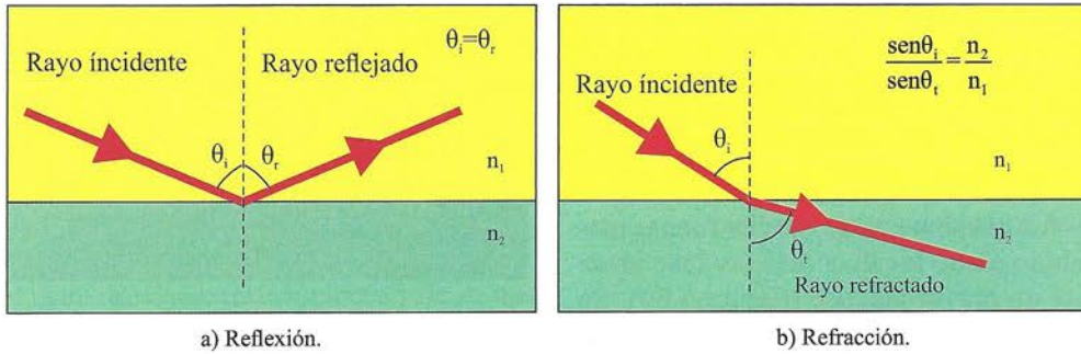
Figura 6.62. Fenómenos ópticos producidos en la fibra óptica.
