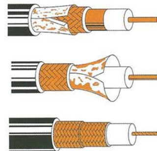
Figura 6.8. Diferentes estructuras de los cables coaxiales.
