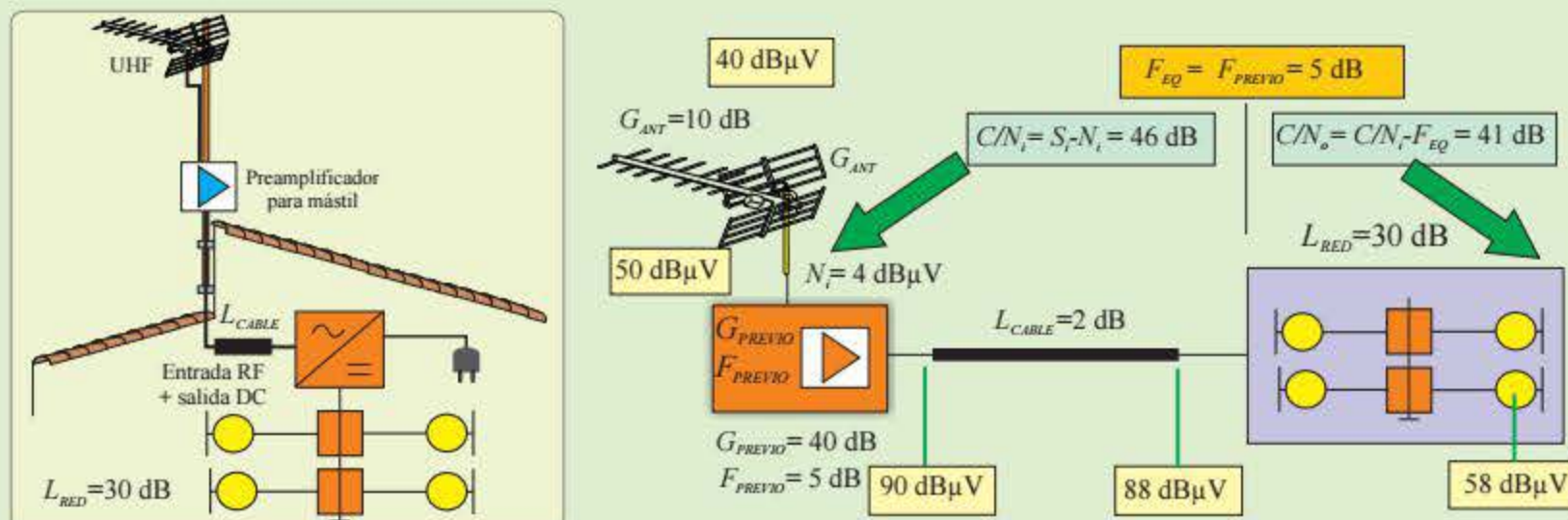
Figura 4.27. Utilización de un preamplificador.
