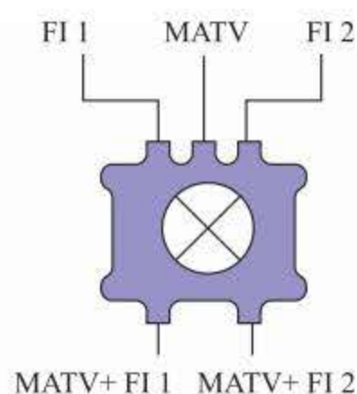
Figura 4.48. Mezclador-repartidor de ICT.
