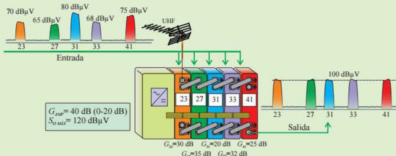
Figura 4.35. Ecualización mediante amplificadores monocanal.
