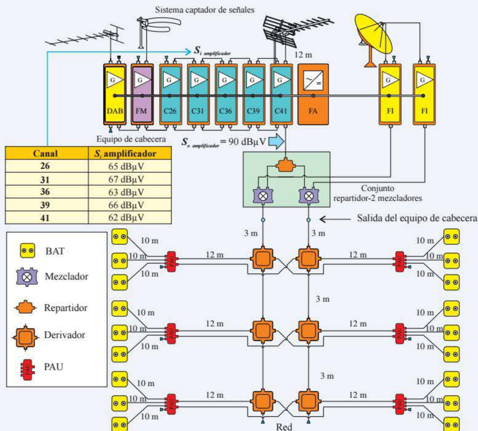
Figura 4.61. Esquema de la red de la ICT de TV.
