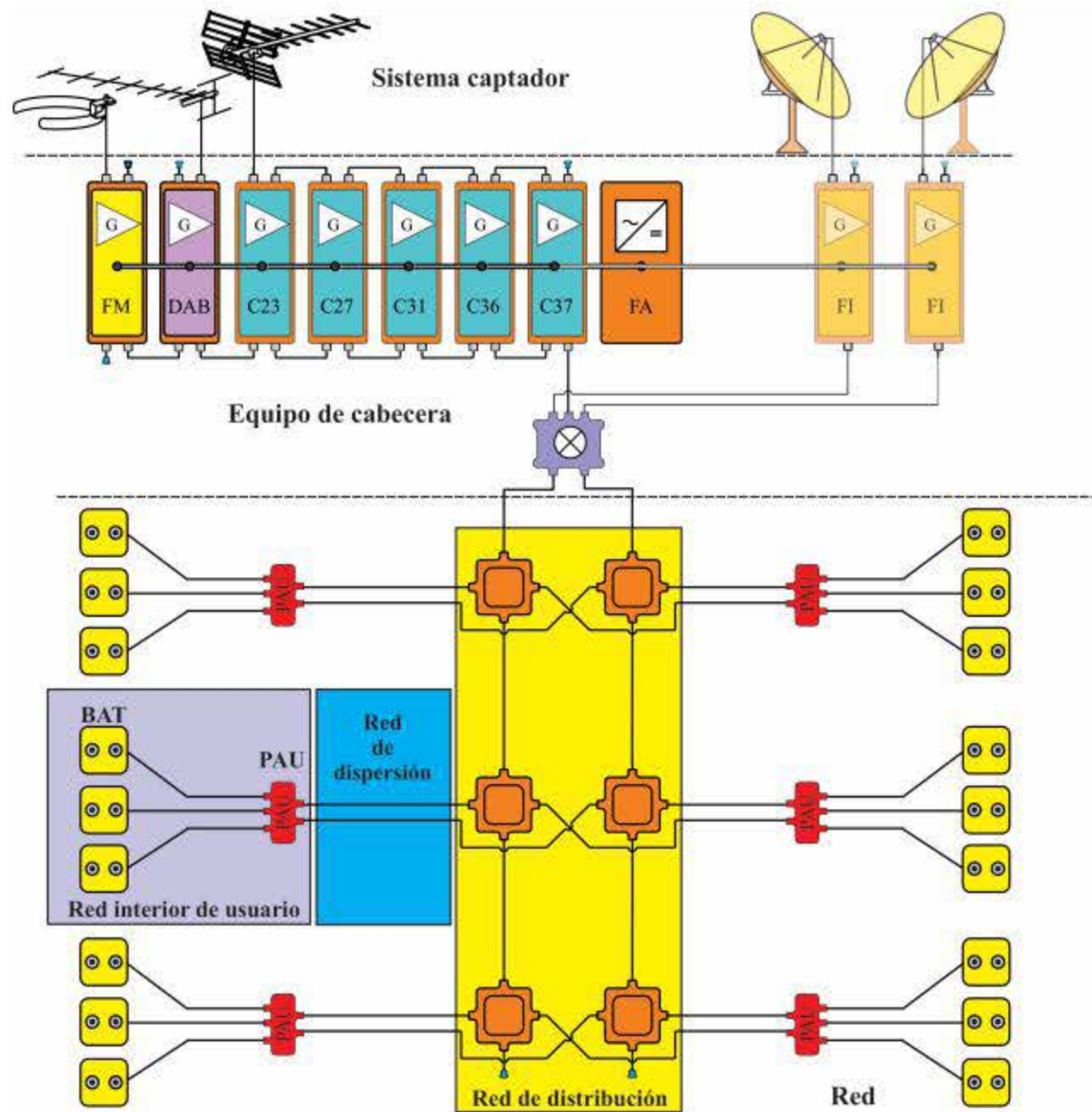
Figura 4.45. Partes que componen la red de televisión.
