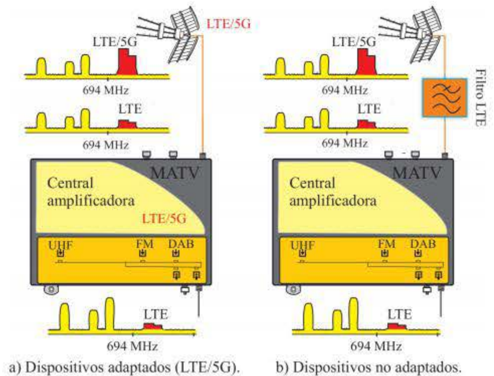
Figura 4.10. Interferencias LTE.
