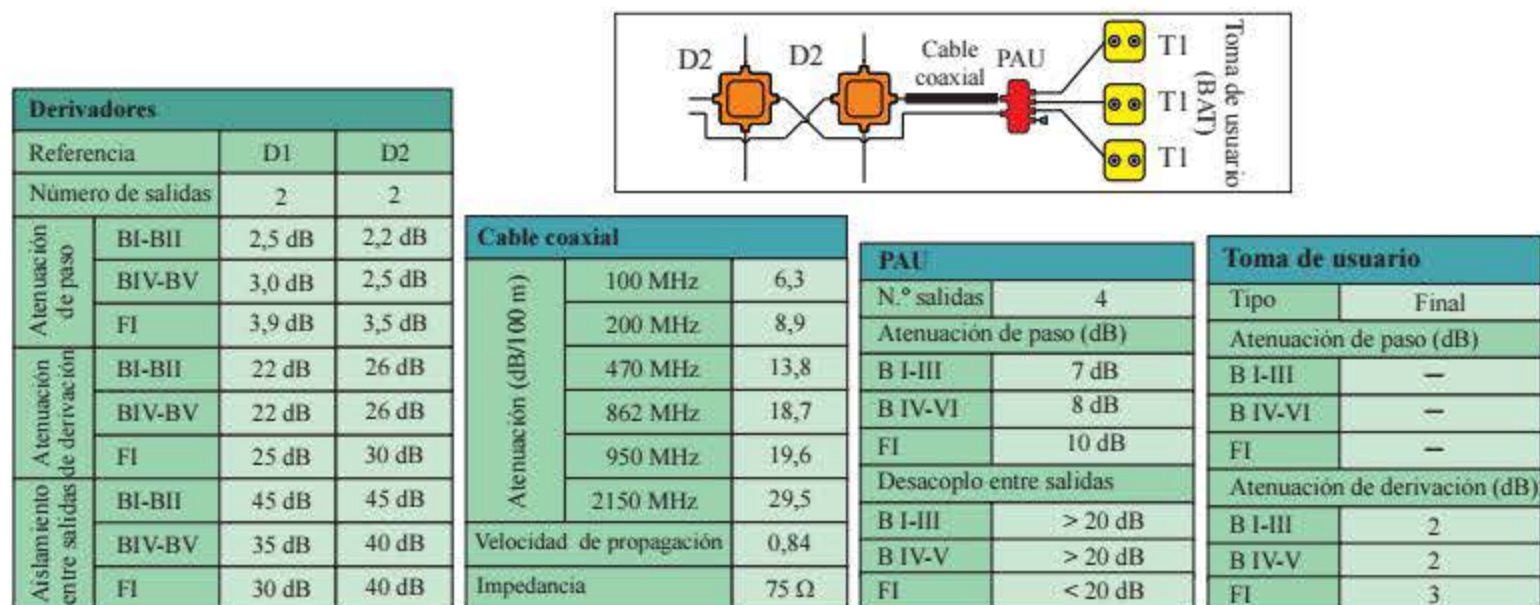
Figura 4.56. Características de los materiales utilizados. Red.
