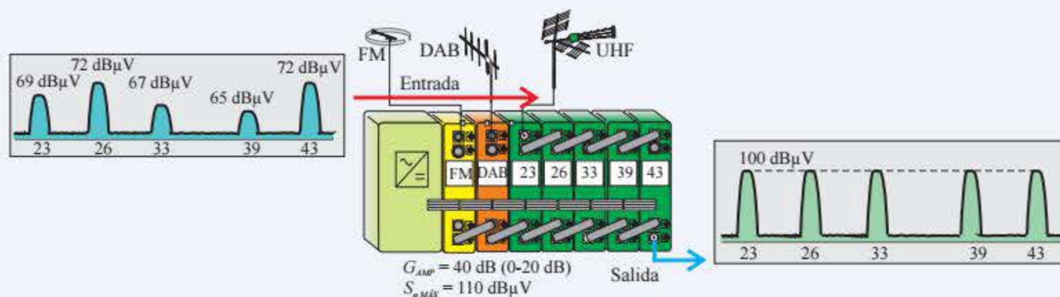
Figura 4.66. Amplificación de canales.
