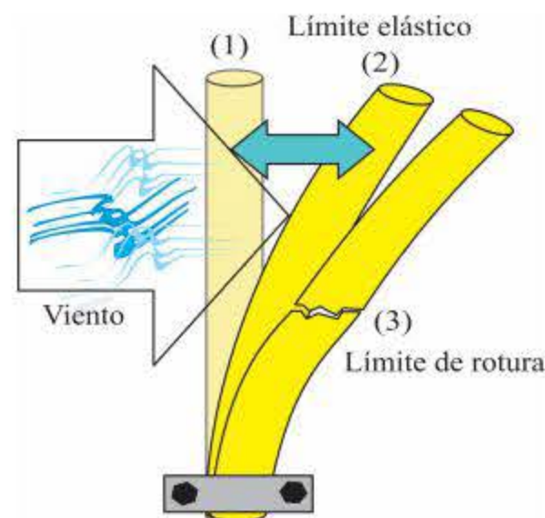
Figura 4.22. Comportamiento del mástil ante el efecto del viento.
