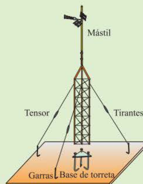
Figura 4.19. Ejemplo de instalación de una torreta.
