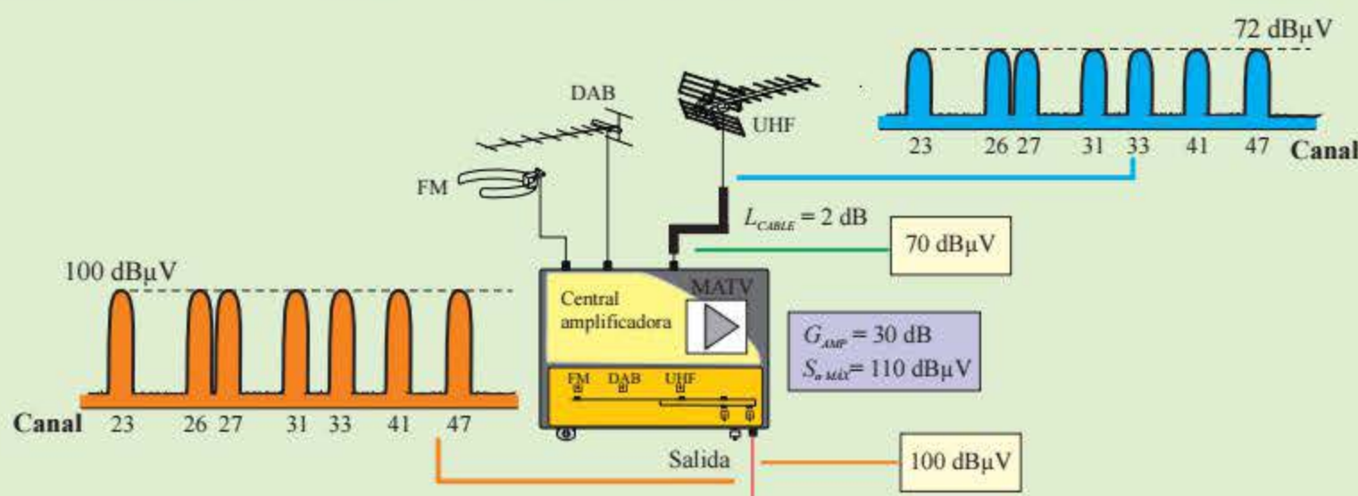
Figura 4.31 Amplificación de canales ecualizados.
