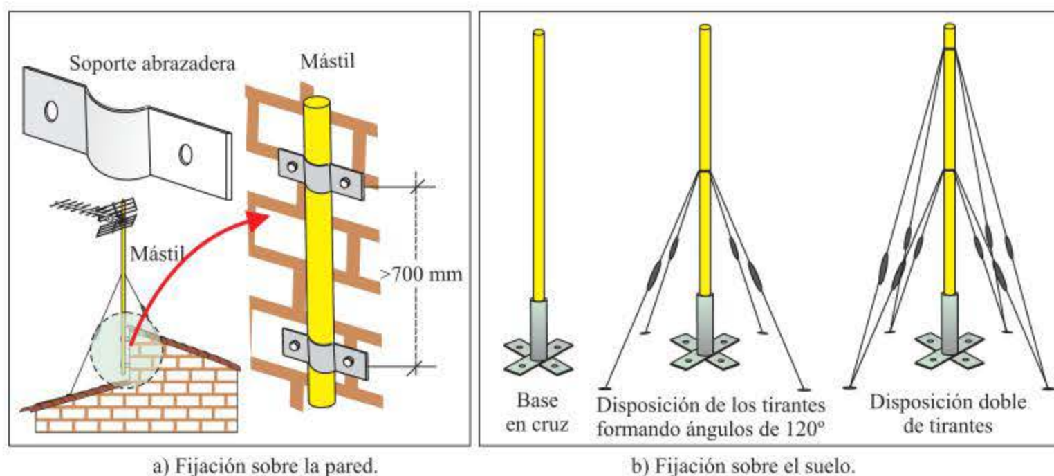
Figura 4.17. Fijación del mástil.
