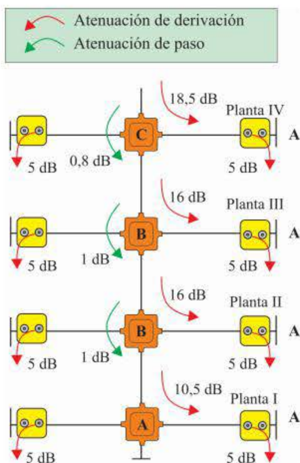
Figura 4.43. Ejemplo de distribución mediante derivadores.
