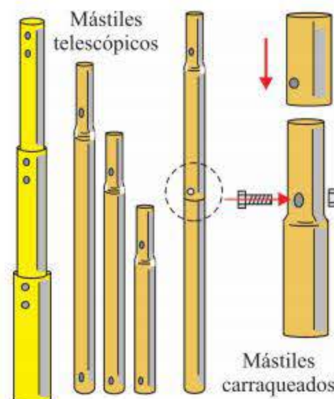
Figura 4.14. Tipos de mástiles.
