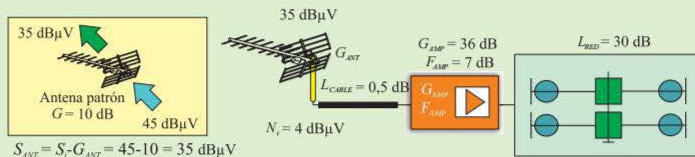
Figura 4.28. Elección de la ganancia de la antena.
