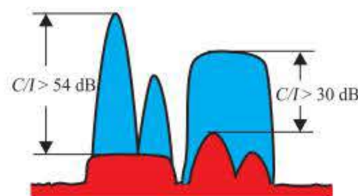
Figura 4.3. Efecto de la intermodulación.
