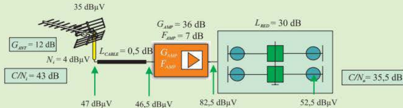
Figura 4.29. Niveles de señal en la red.
