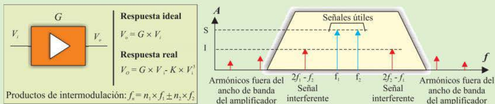
Figura 4.2. Prueba de dos tonos.
