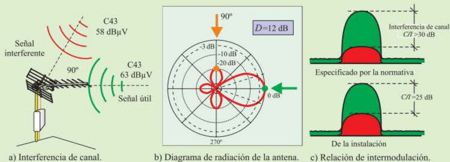
Figura 4.11. Ejemplo de interferencia de canal.
