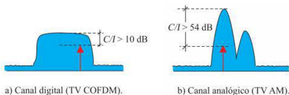
Figura 4.5. Relación portadora/interferencia a frecuencia única.
