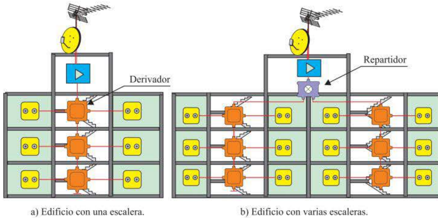
Figura 4.42. Tipos de edificios.
