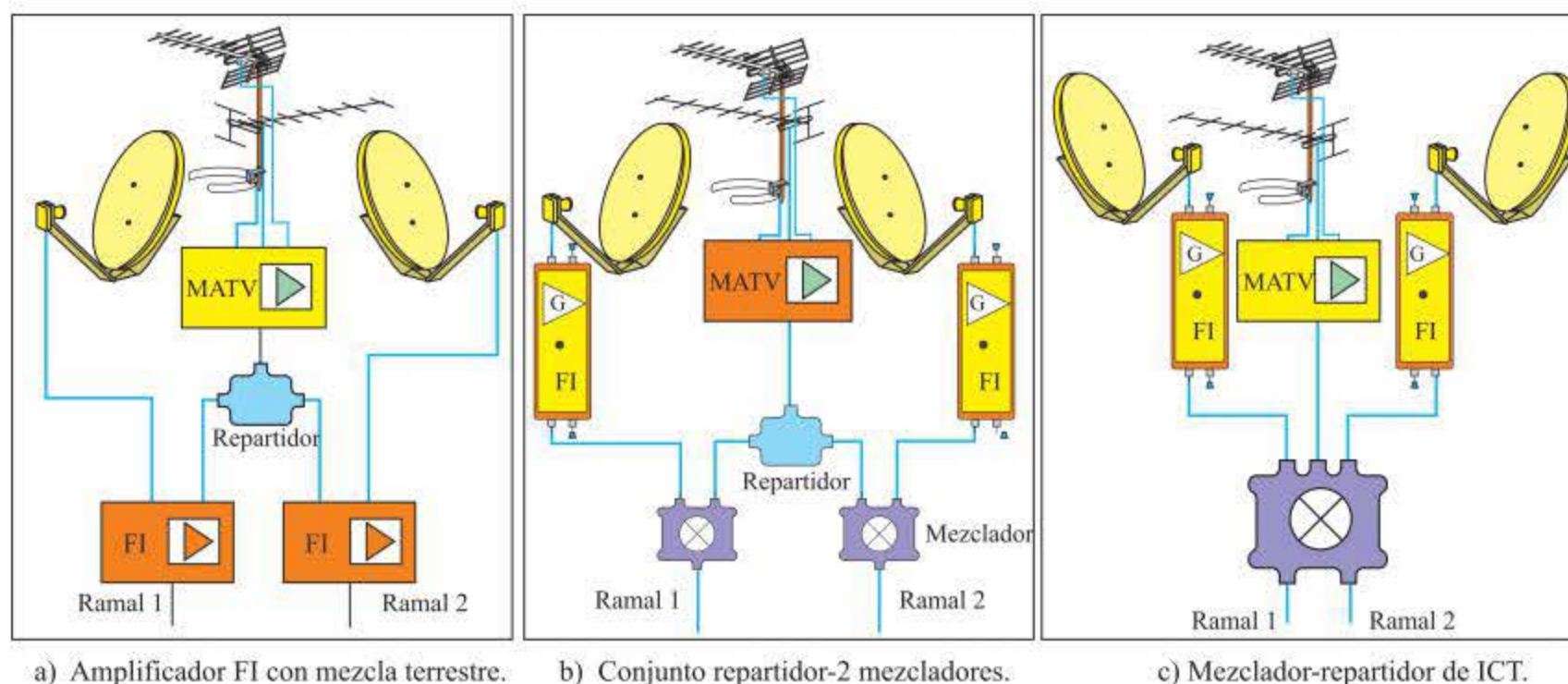
Figura 4.47. Mezcla de las señales satélite y terrestre en una distribución a dos hilos.
