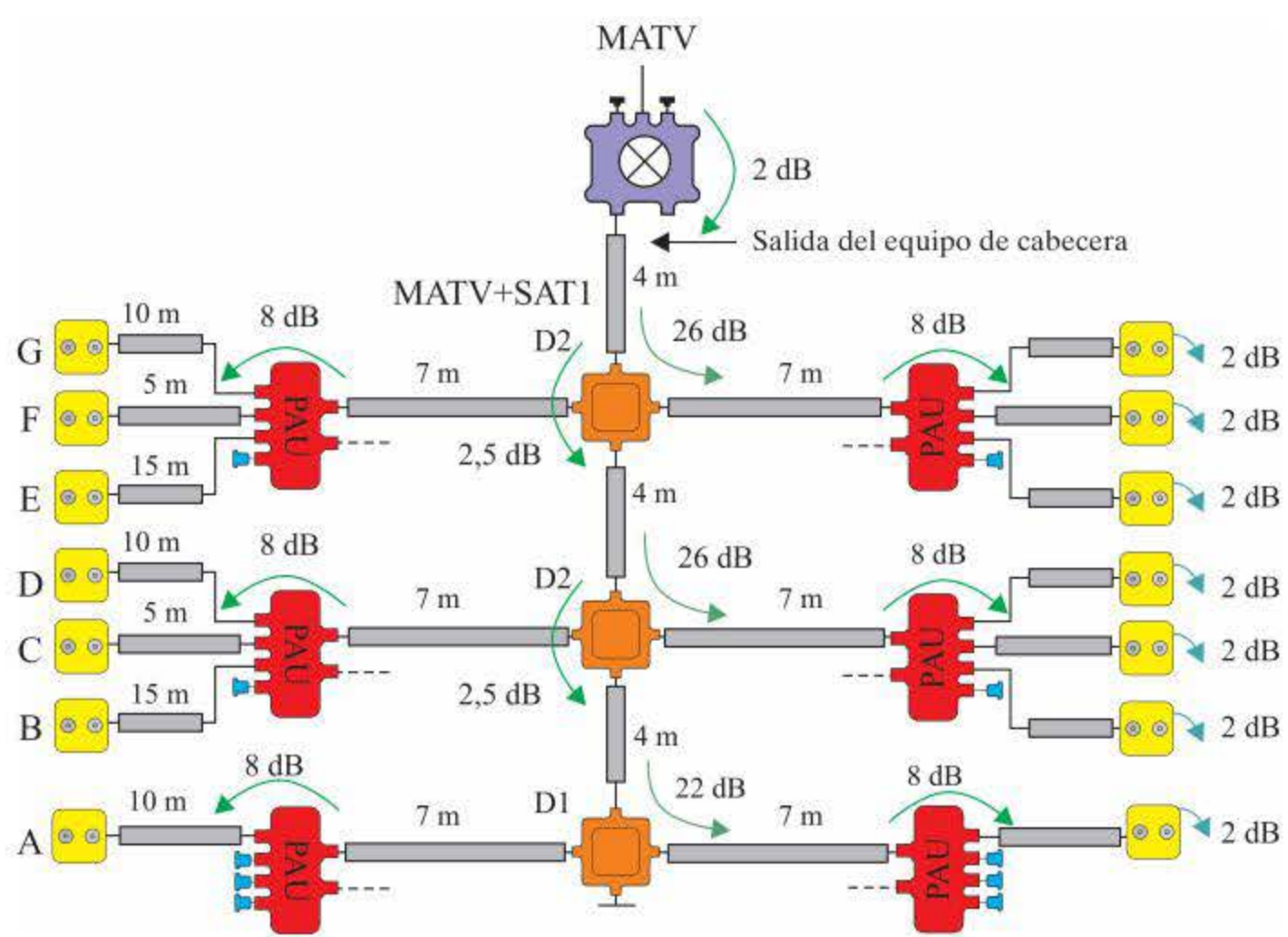
Figura 4.57. Análisis de las pérdidas de la red para la banda de UHF.
