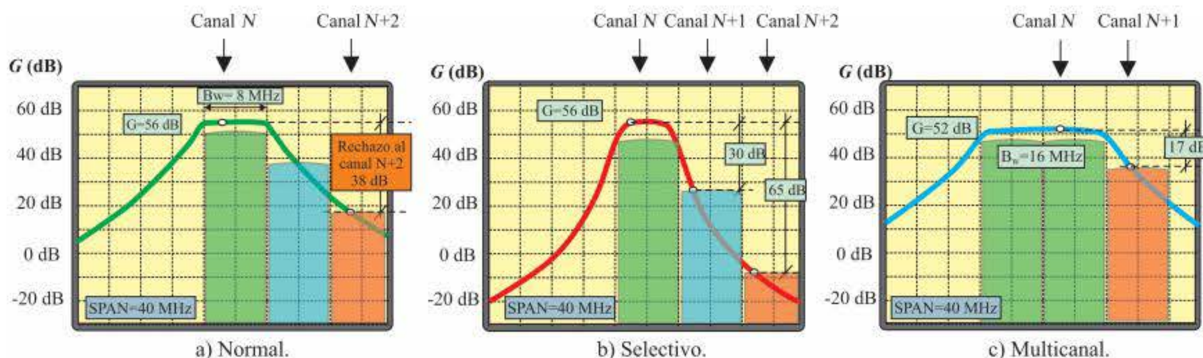
Figura 4.37. Respuesta en frecuencia de un amplificador monocanal.
