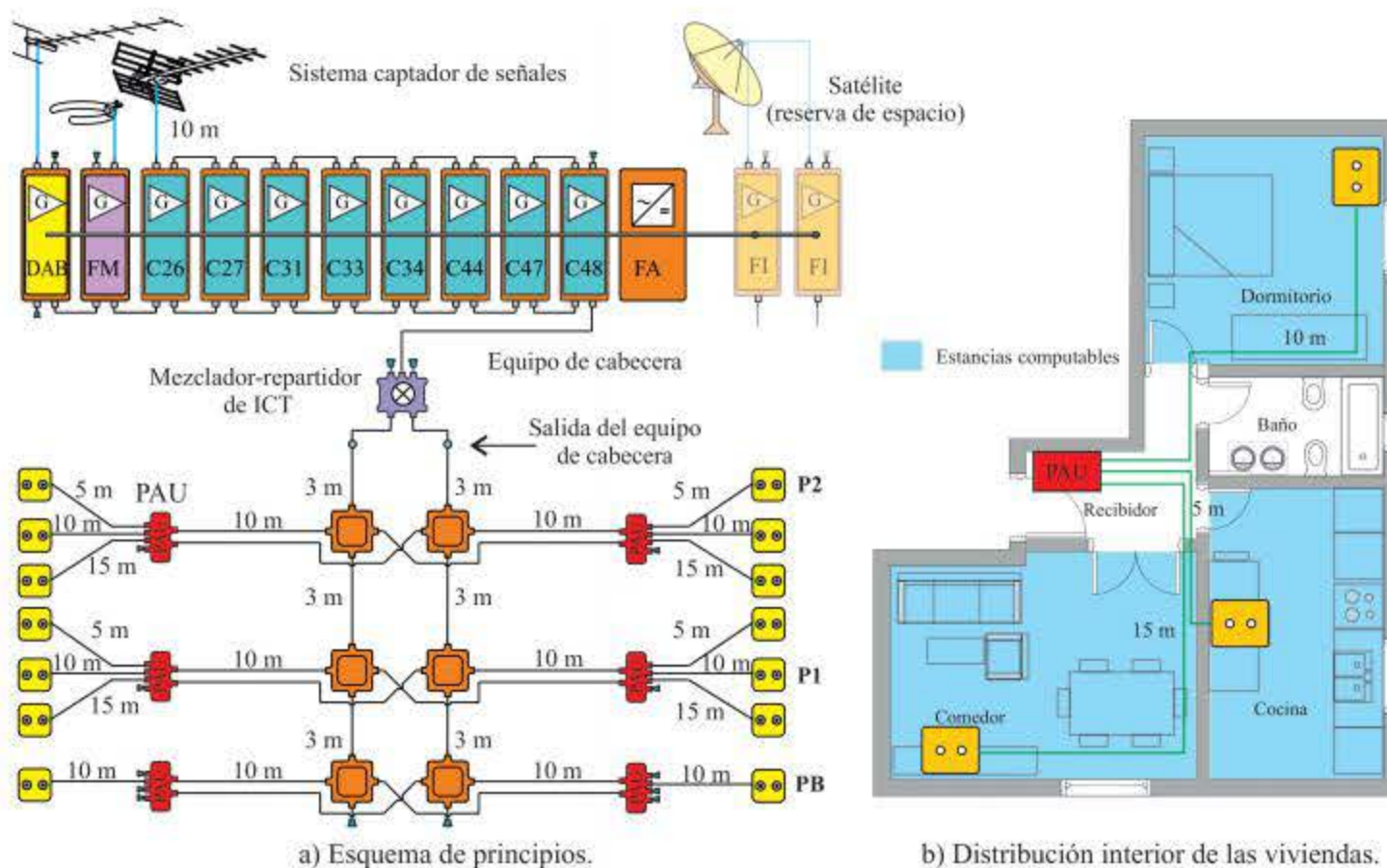
Figura 4.53. Edificio de la instalación ICT.
