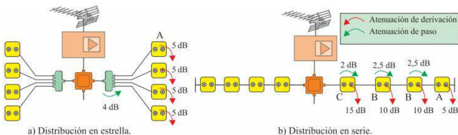
Figura 4.44. Red interior de usuario.
