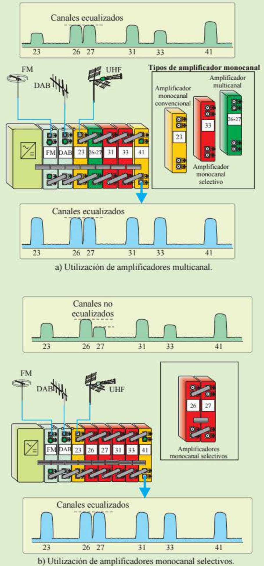
Figura 4.39. Amplificación de canales adyacentes.
