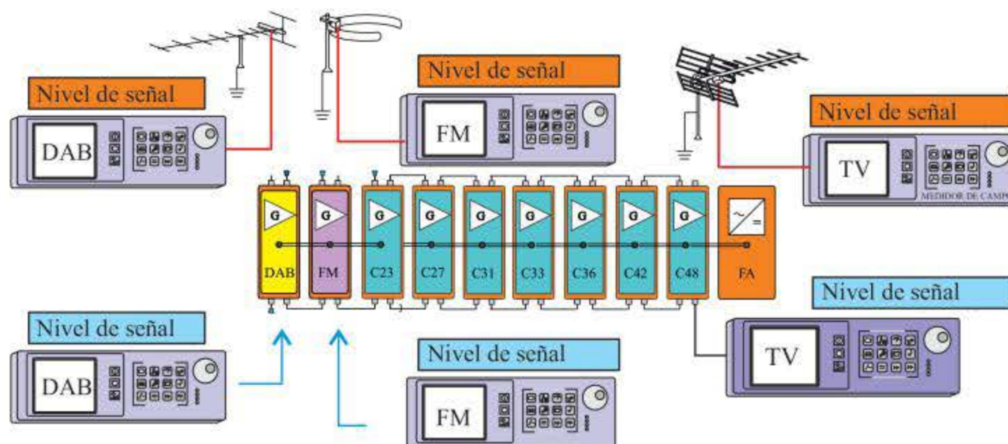
Figura 4.59. Medida de las señales de radiofrecuencia en la salida y entrada de los amplificadores.
