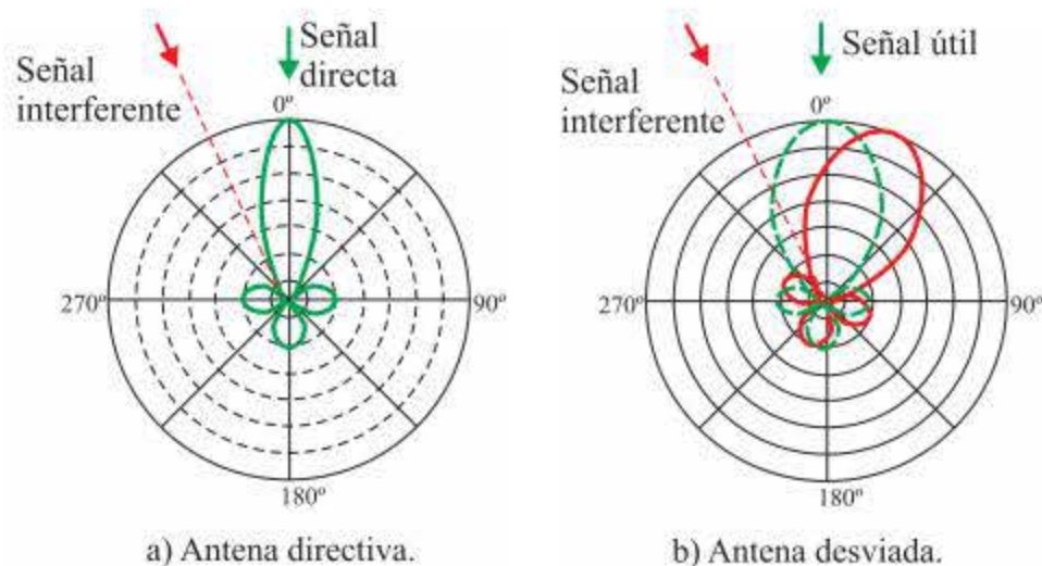
Figura 4.9. Soluciones a las interferencias.
