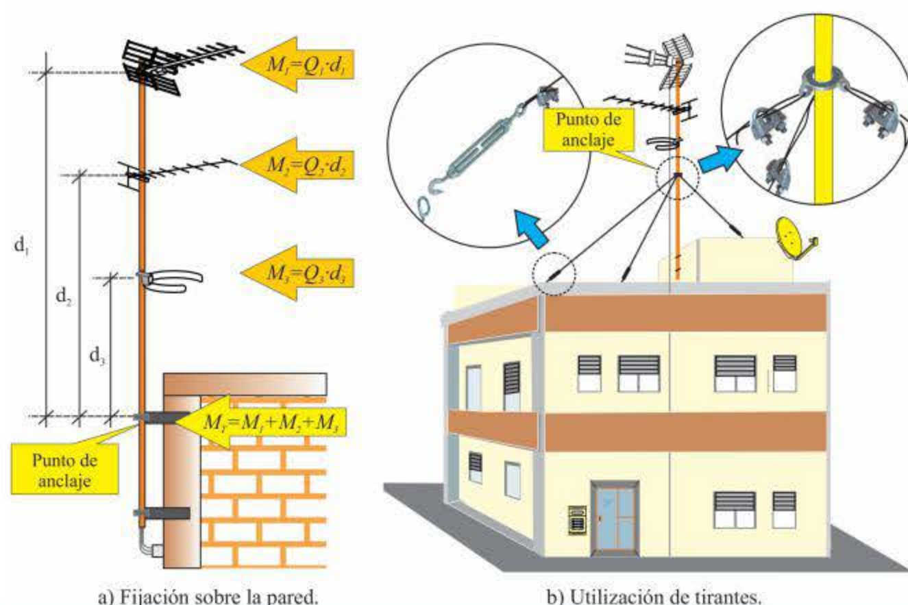
Figura 4.23. Cálculo del momento flector.
