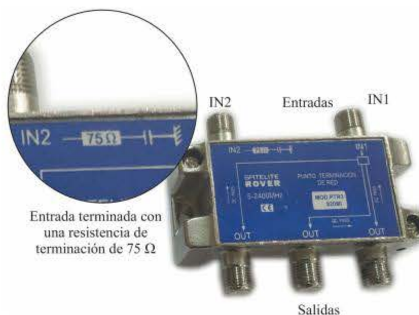
Figura 4.50. Ejemplo de PAU de una instalación de TV.
