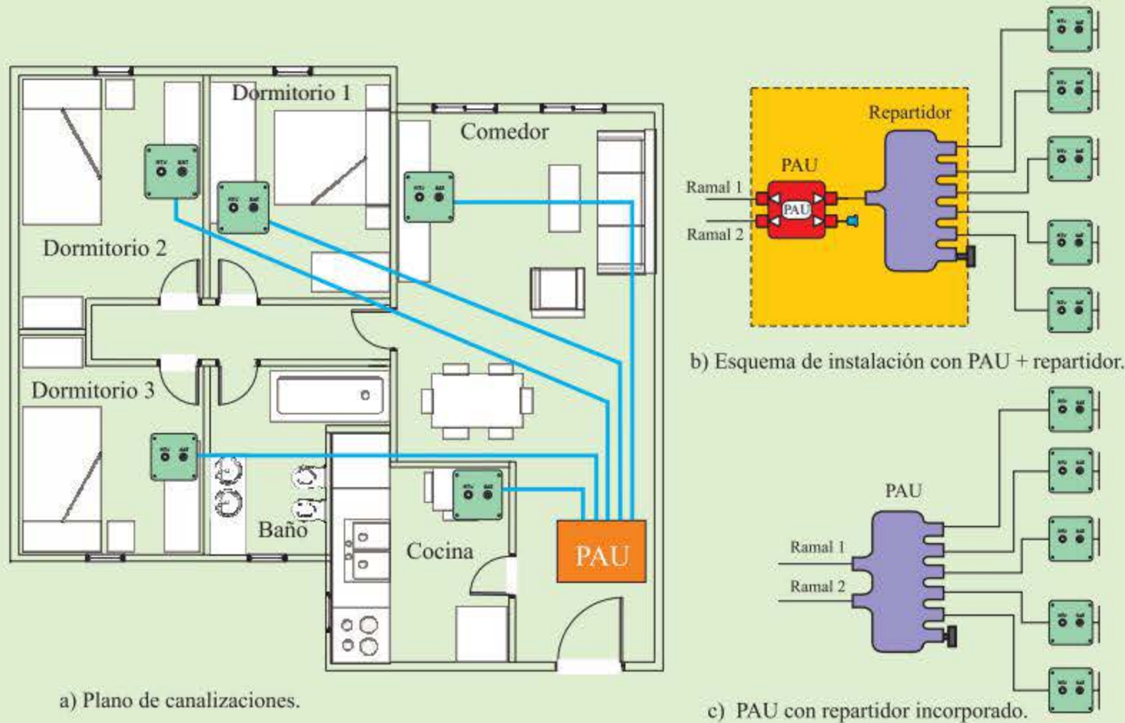
Figura 4.52. Instalación interior de usuario.
