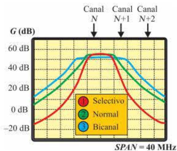
Figura 4.36. Comparación entre diferentes amplificadores selectivos.
