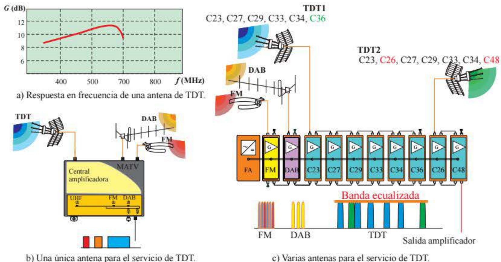
Figura 4.7. Antenas de TDT.
