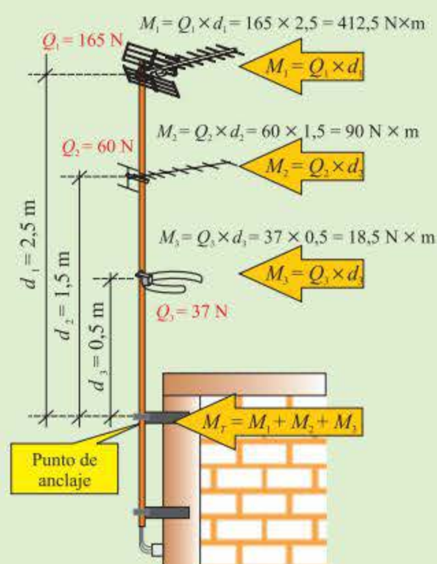
Figura 4.24. Ejemplo de cálculo del momento flector.
