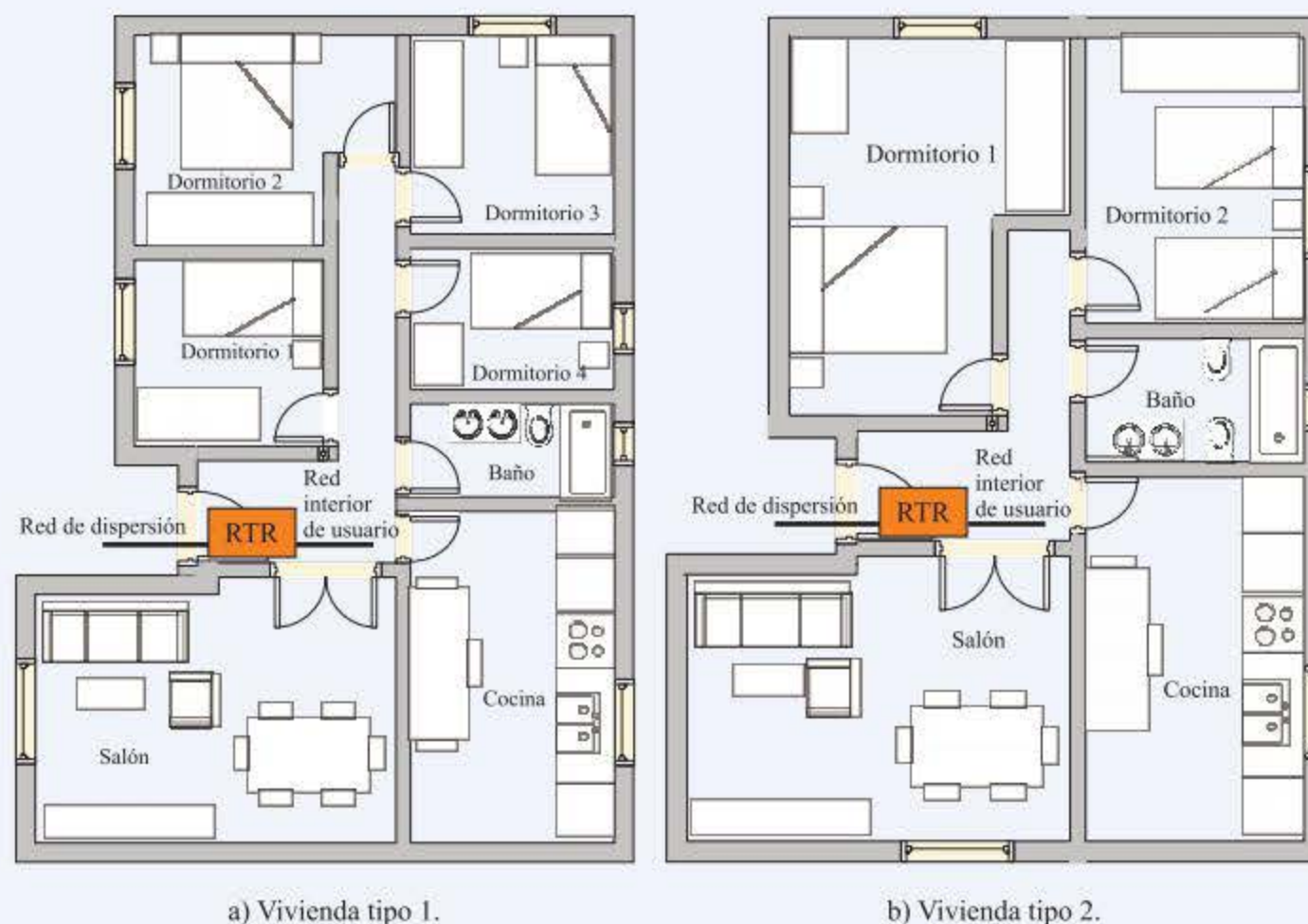
Figura 4.62. Plano de la instalación interior de usuario.
