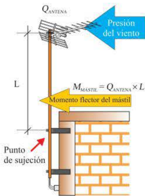
Figura 4.21. Momento flector de un mástil.
