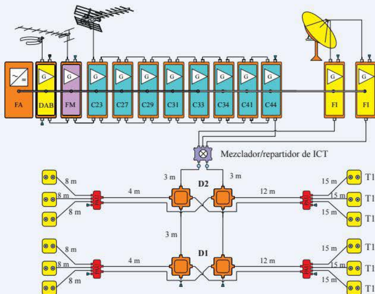
Figura 4.63. Instalación de distribución de la señal de TV de una ICT.
