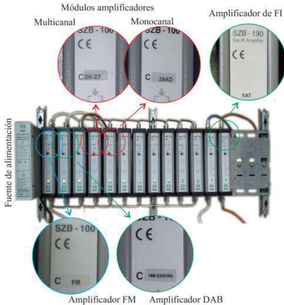
Figura 4.38. Tipos de amplificadores.
