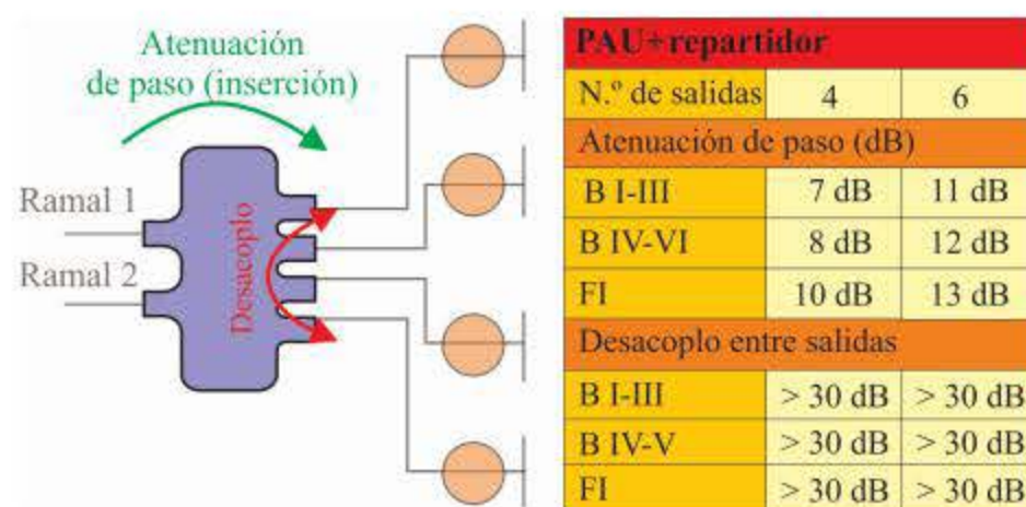
Figura 4.51. Características técnicas de un PAU.
