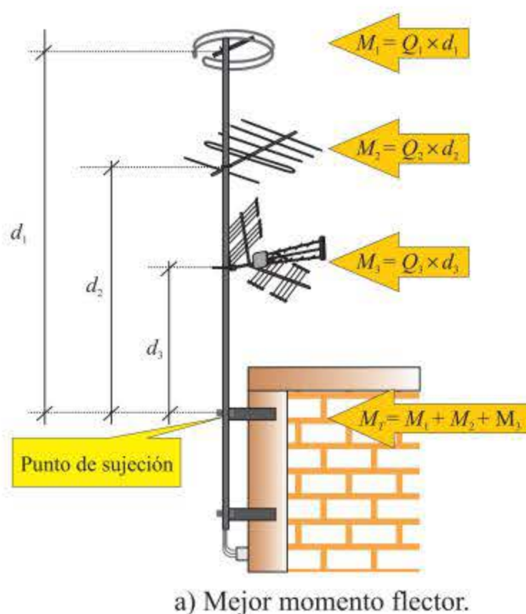
Figura 4.25. Criterios de instalación de las antenas sobre el mástil.
