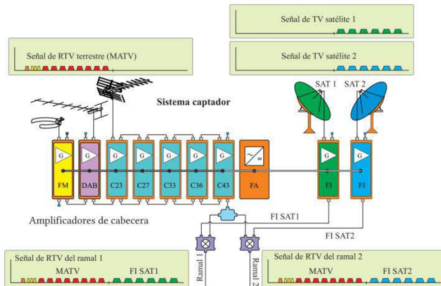
Figura 4.46. Distribución de señales en los ramales.
