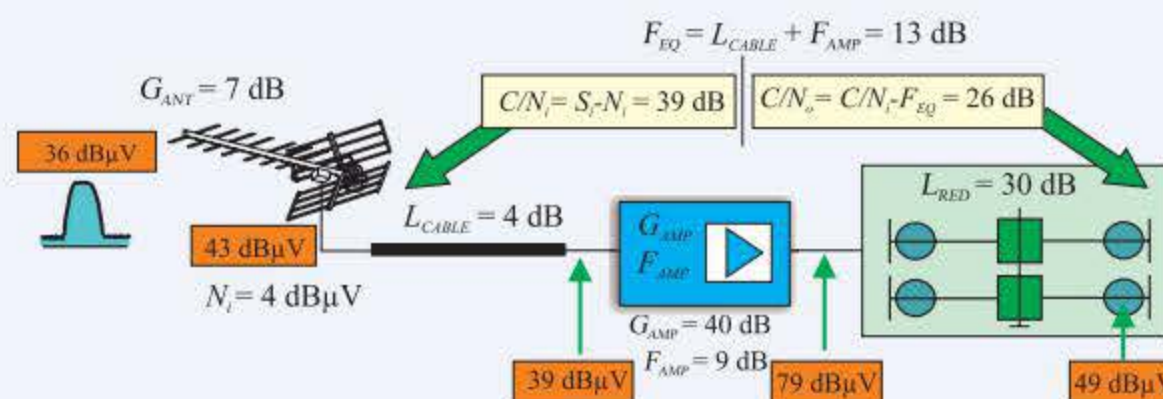
Figura 4.67. Instalación con preamplificador.
