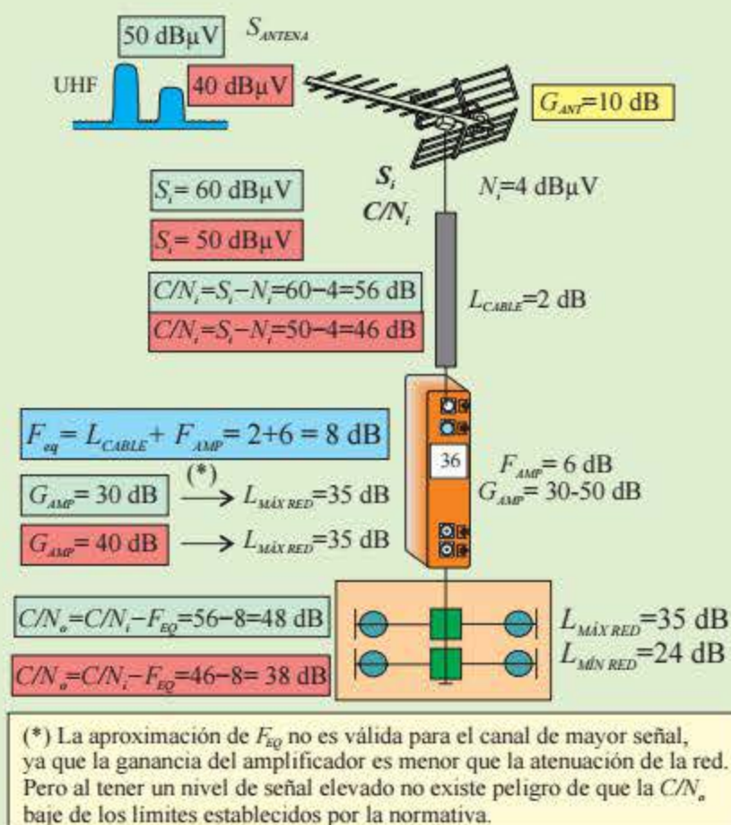
Figura 4.41. Evaluación de la C/N de salida.
