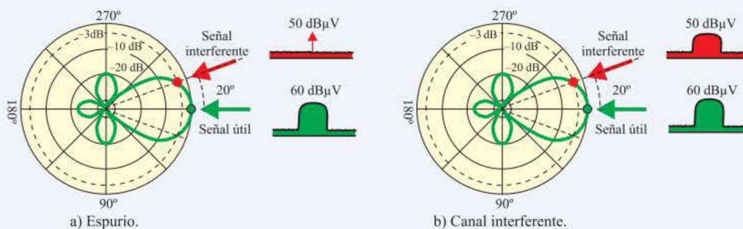
Figura 4.65. Interferencia.
