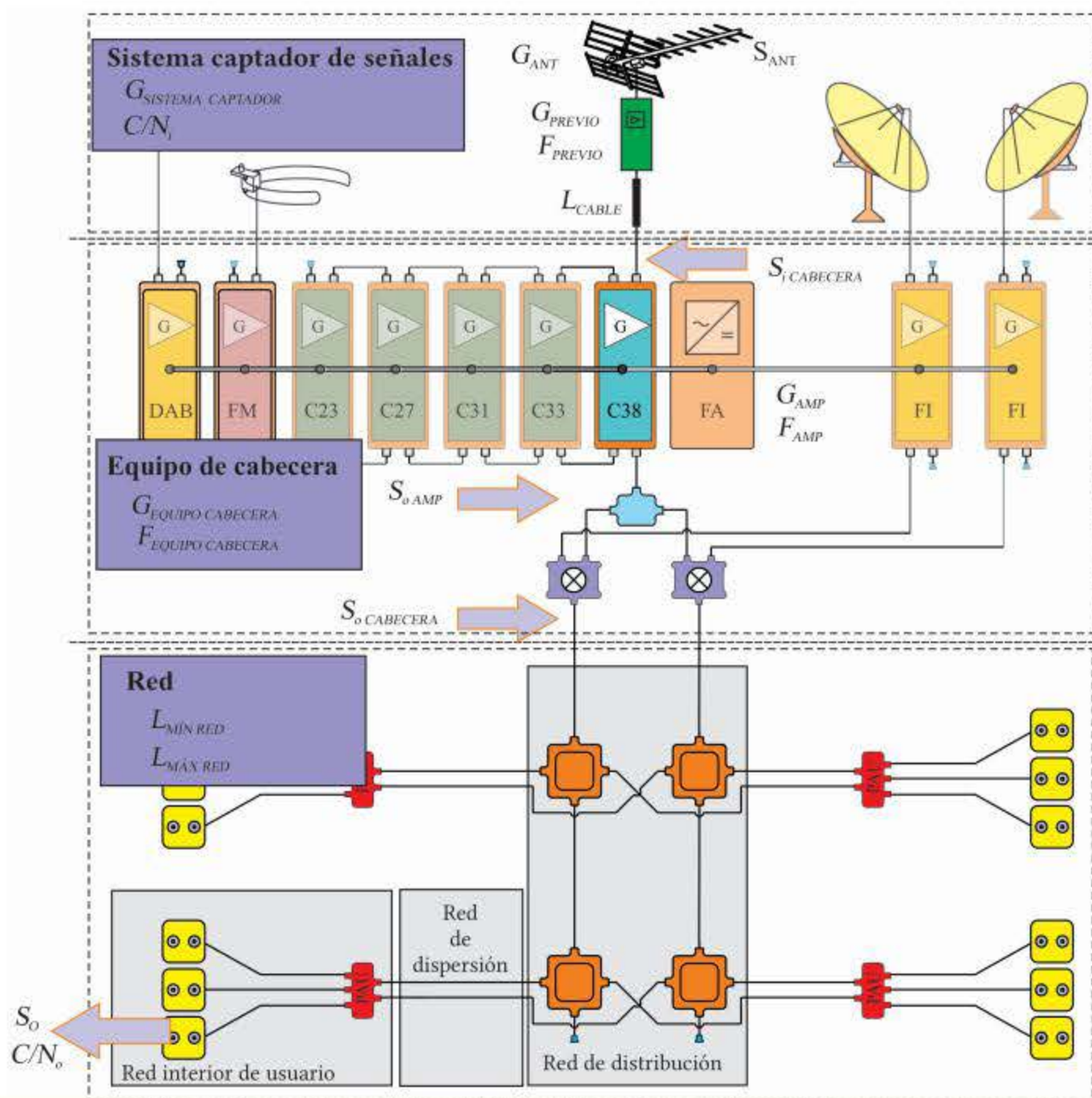
Figura 4.6. Diseño de una instalación.
