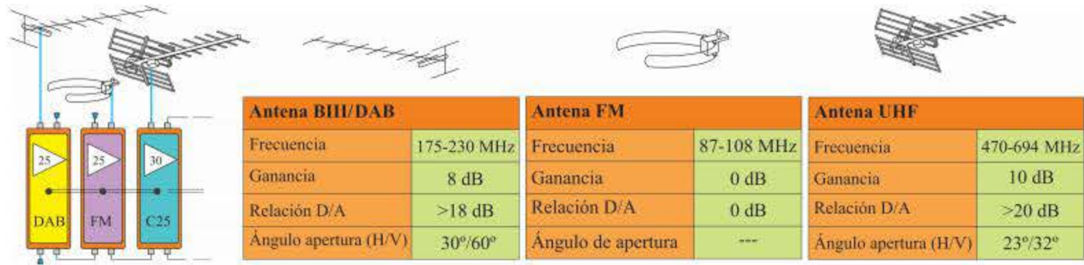
Figura 4.54. Características del sistema captador.
