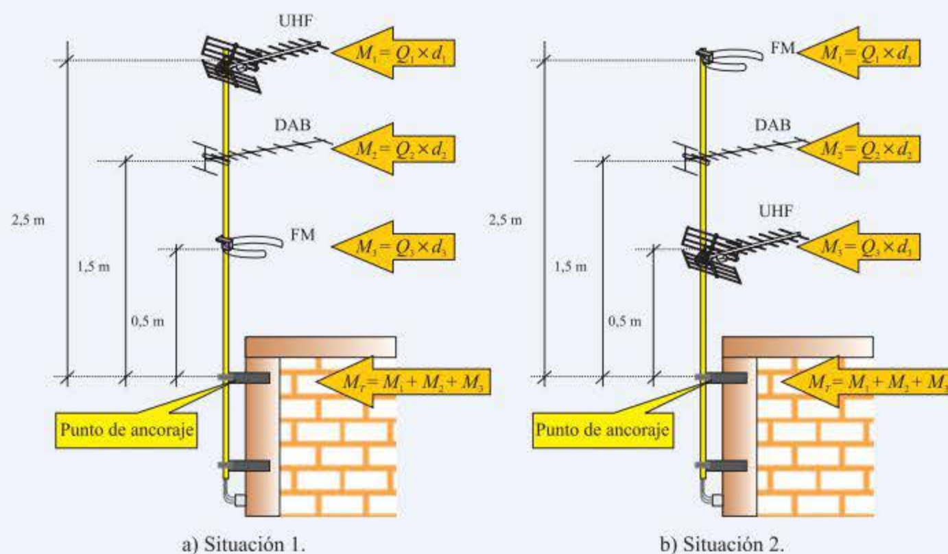
Figura 4.64. Cálculo del momento flector del mástil.
