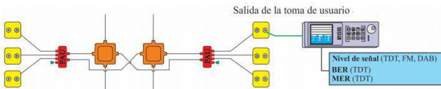
Figura 4.60. Medida de la calidad en la toma de usuario.
