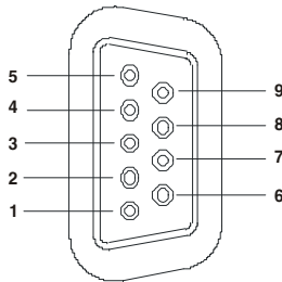
Figura 42.- Conector RS-232C. Vista exterior.
