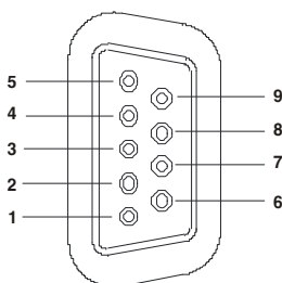
Figure 42.- Connecteur RS-232C. Raccordements vus de face.
