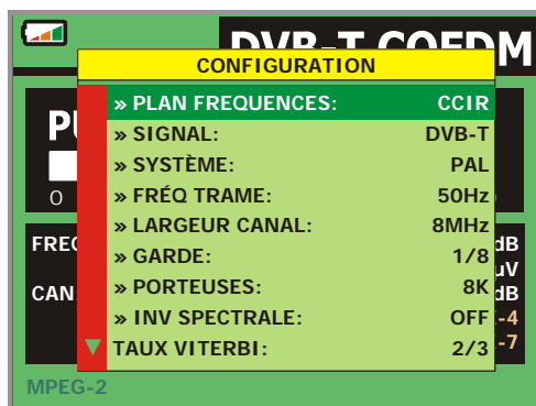
Figure 19.- Écran de configuration de mesure de signaux modulés en COFDM.
