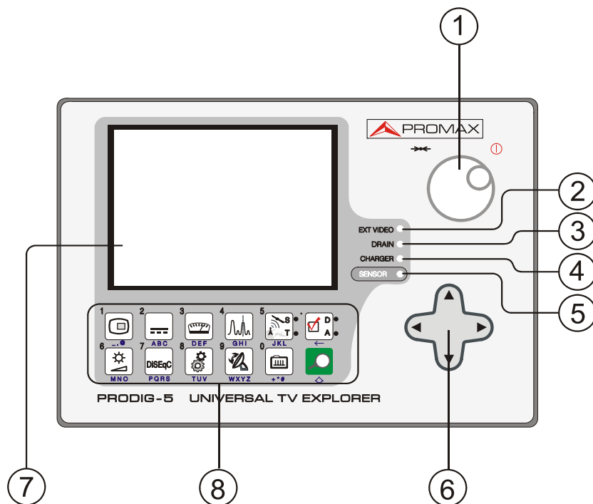
Figure 3.- Panneau frontal.
