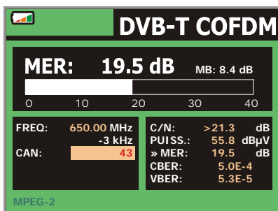
Figure 34.- Écran de mesure du MER pour signaux DVB-T modulés en COFDM .
