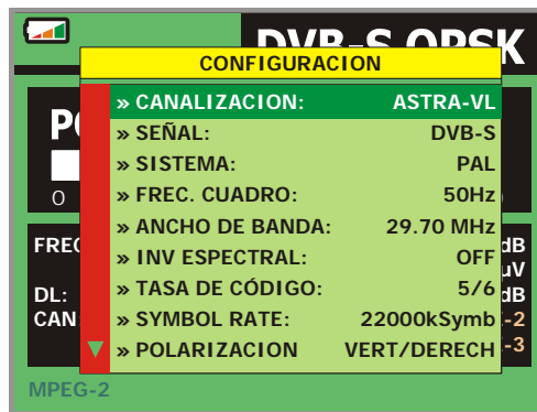
Figura 20.- Pantalla de configuración de medida de señales moduladas en QPSK.
