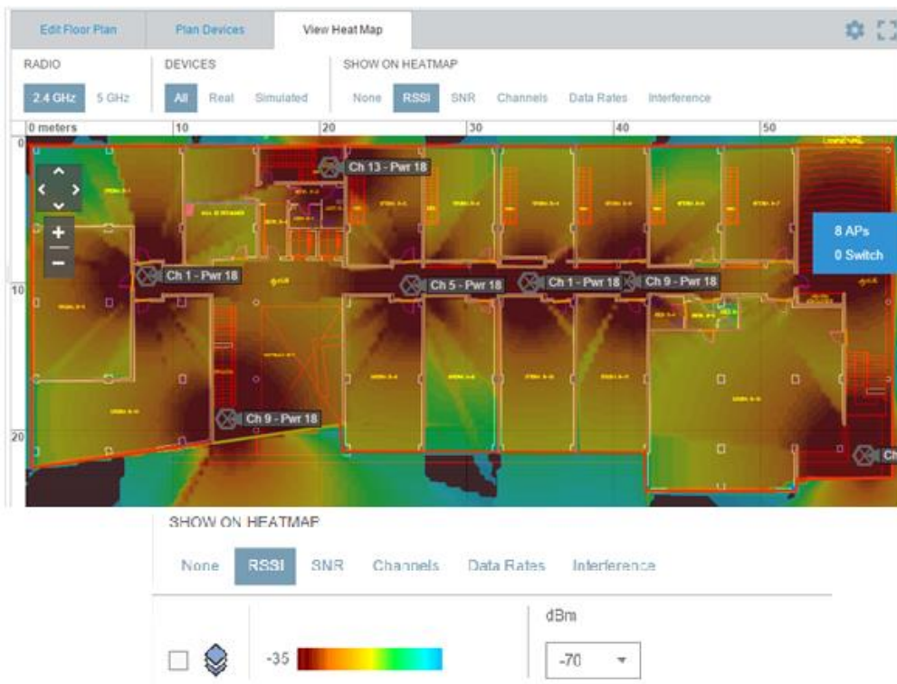
Figura 4-11. Nivel de señal a 2.4 GHz en la planta baja
