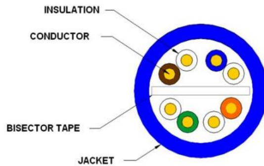
Figura 6-1. Sección transversal del cable de pares
